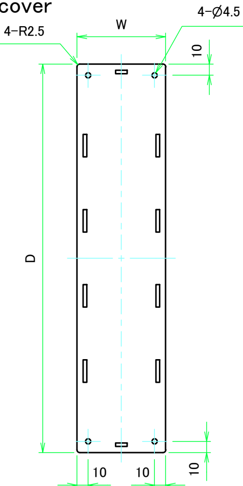
上カバー表面 / Top cover Frontside
