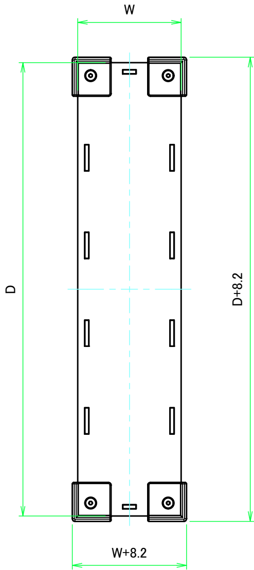
上カバー / Top cover
